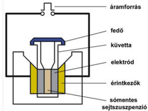
6.17. Ábra Az elektroporátor készülék képe, valamint a kísérlet elvi felépítése.
