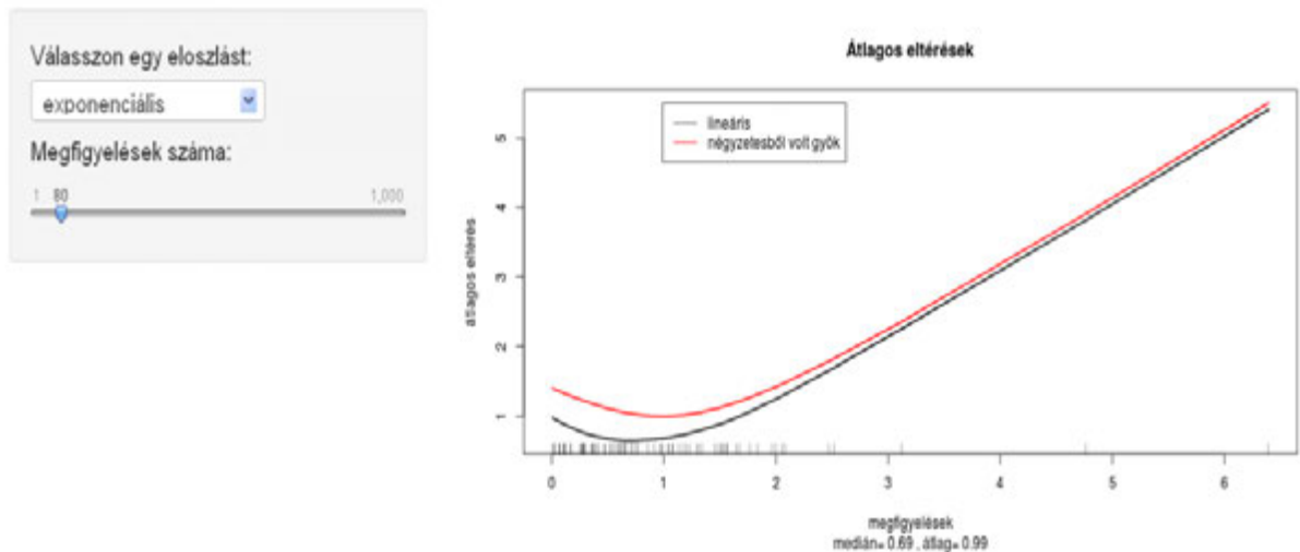
11.7. ábra. Az átlag és a medián optimumtulajdonsága az exponenciális eloszlásra 80 elemű mintára
