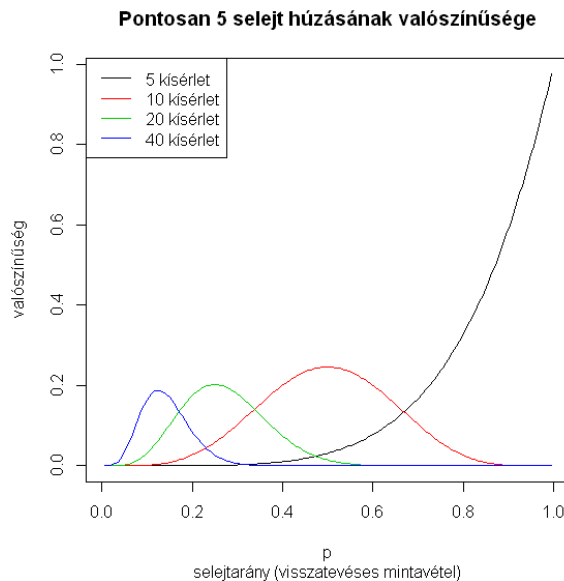
3.9. ábra. Pontosan 5 selejtes húzásának valószínűsége a kísérletek számának és a p -nek a függvényében, a visszatevées mintavételnél 11.14 kód
