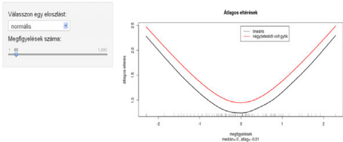
11.6. ábra. Az átlag és a medián optimumtulajdonsága a normális eloszlásra 80 elemű mintára
