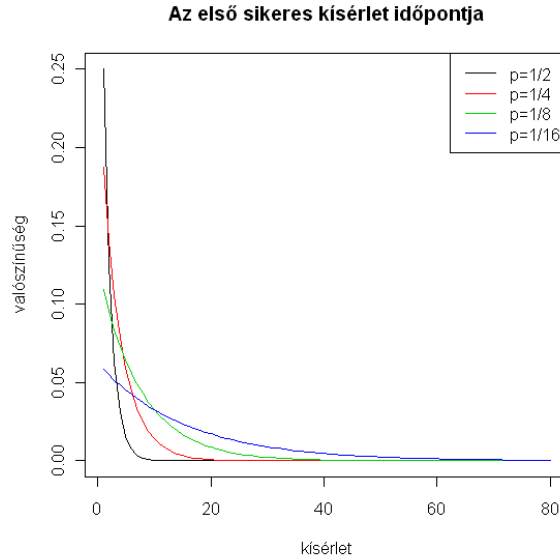
3.14. ábra. Az első sikeres kísérlet sorszámanak eloszlása különböző p -re, 11.18 kód
