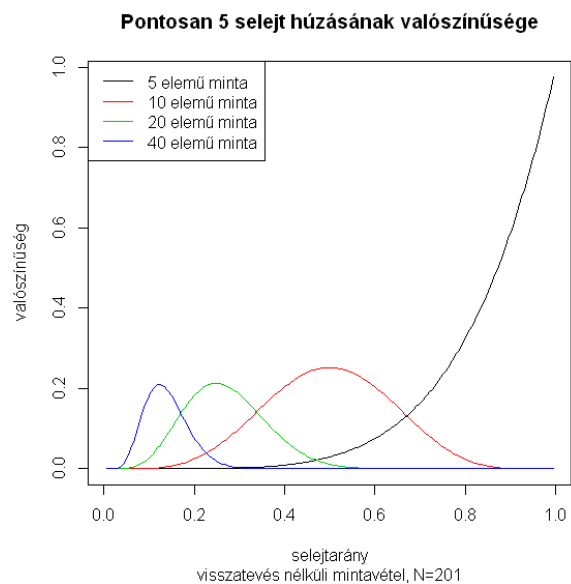
3.10. ábra. Pontosan 5 selejtes termék húzásának valószínűsége a minta elemszámának és a sokaságban levő selejtesek számának a függvényében, N=201 , 11.15 kód
