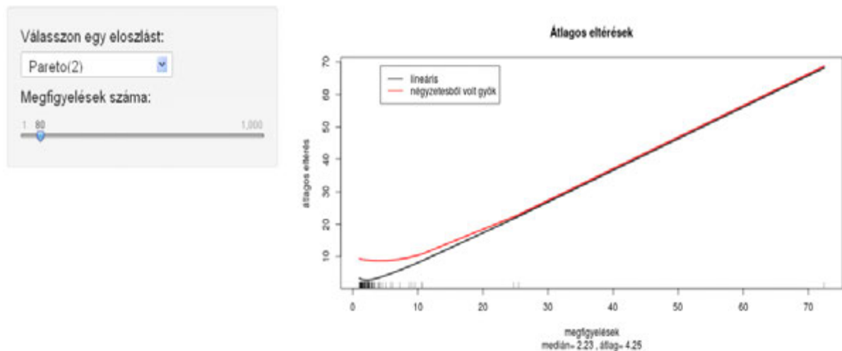
11.8. ábra. Az átlag és a medián optimumtulajdonsága a Pareto(2) eloszlásra 80 elemű mintára
