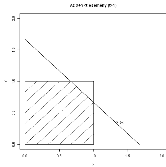
5.8. ábra. 2 koordináta összege
