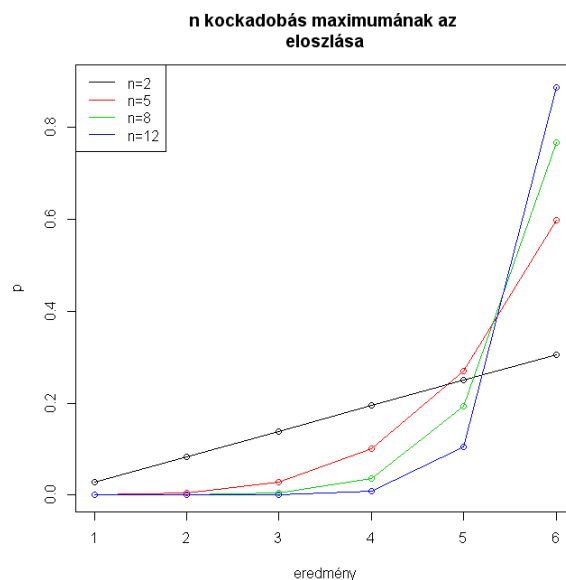
2.5. ábra. A legnagyobb dobott szám eloszlása különböző kocka-számokra (2.9 feladat)
