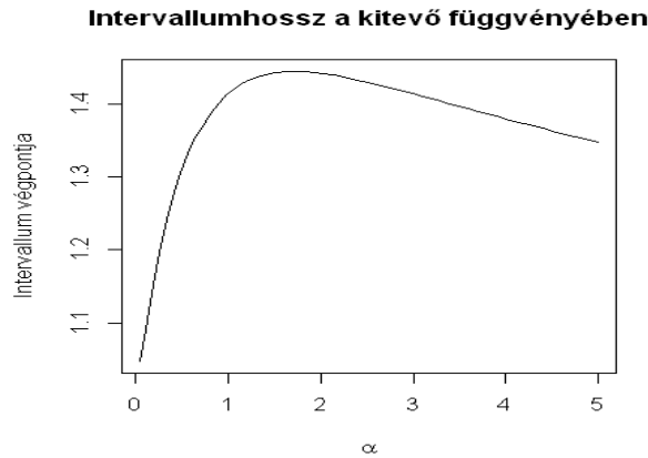
5.6. ábra. Intervallumhossz különböző kitevőjű sűrűségfüggvények esetében
