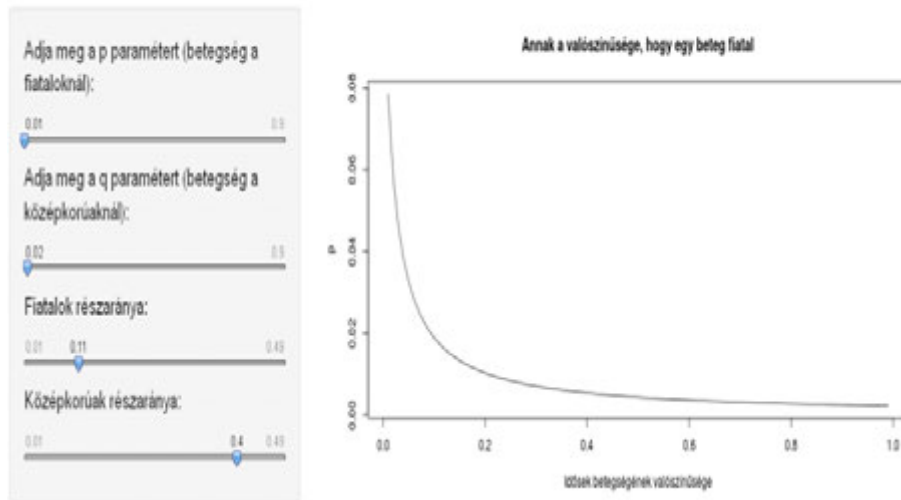
11.2. ábra. A (3.12) példa valószínűségének függése az idők megbetegedési valószínűségétől, az ábra baloldalán látható paraméterbeállítás mellett, 11.22 kód
