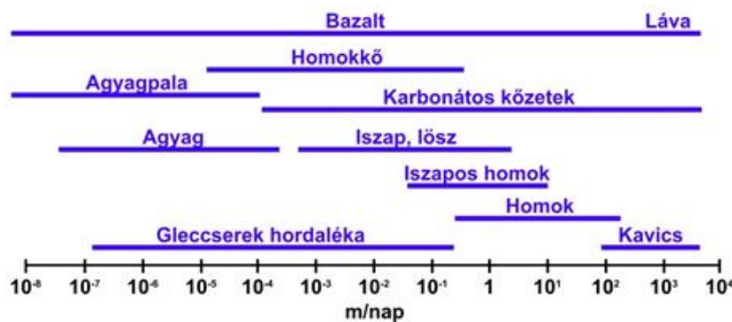
3.15. ábra. Különböző típusú kőzetek és talajok vízvezető-képessége (Heath, 1983 nyomán)
