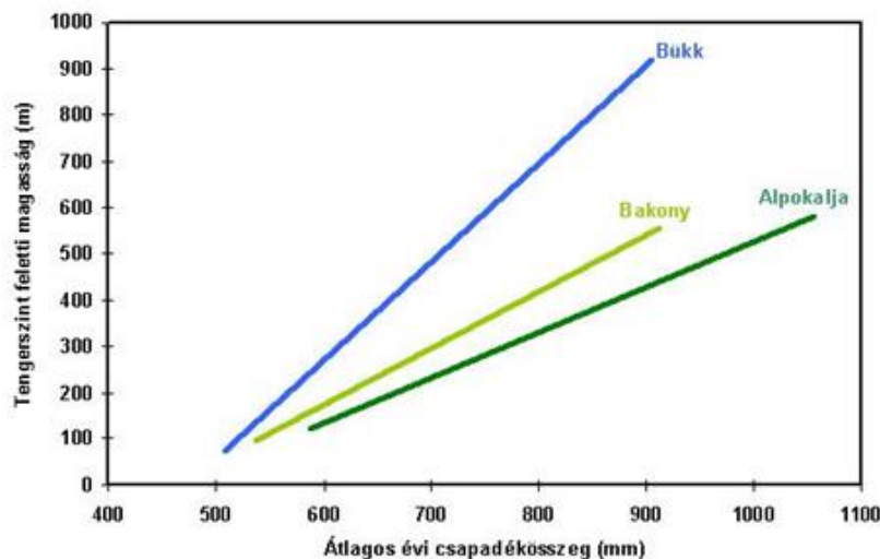
3.11. ábra: A domborzat hatása a csapadékra a hazai középhegységek területein (Stelczer, 2000 nyomán)
