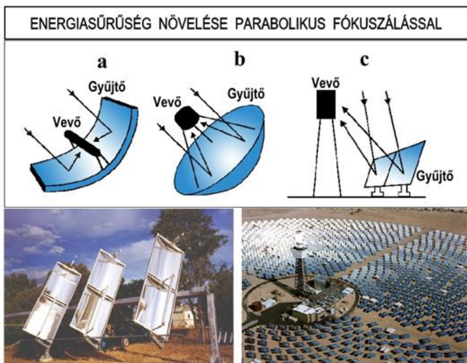
2.7. ábra. Parabolikus tükrörendszerek a gyakorlatban: a. hengeres parabolatükrök, vonalas vevővel; b. parabolafelület, pontszerű vevővel; c. parabolafelületet közelítő síktükrörendszer, toronyvevővel
