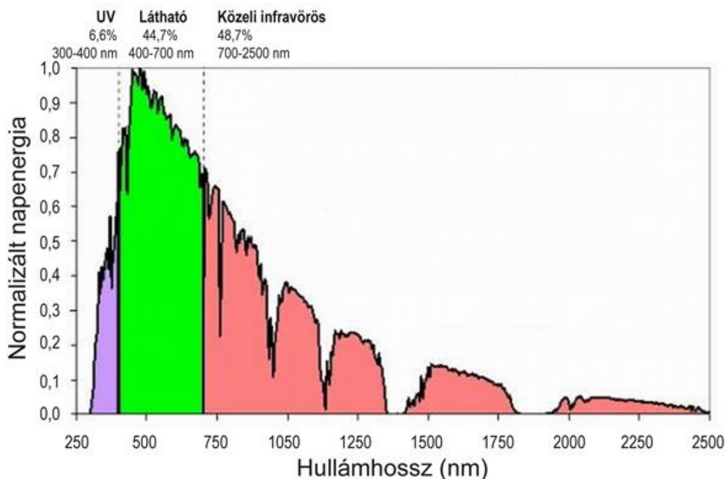
12.7. ábra: A beérkező napsugárzás spektrális eloszlása. A felszínre érkező napenergia csaknem fele a közeli infravörös tartományba esik. A hidegtetők anyaga ebben a tartományban jó visszaverőképeséggel rendelkezik.
