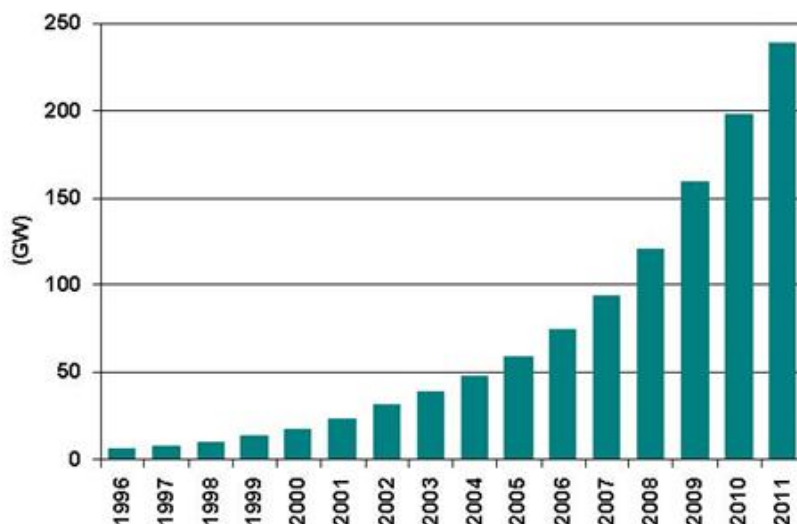
2.12. ábra. A világ szélenergiatarmelésének növekedése az 1996-2011 időszakban (Adatok: GWEC)
