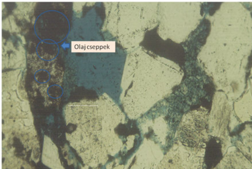
3.11. ábra. Szénhidrogéncseppek elhelyezkedése a nagyobb szemcseközi hézagokban
