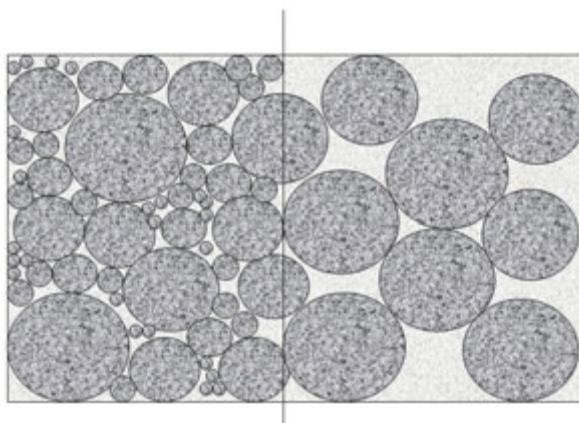
3.2. ábra. Szemcseközi porozitás alakulása különböző szemcseméret-eloszlás esetén
