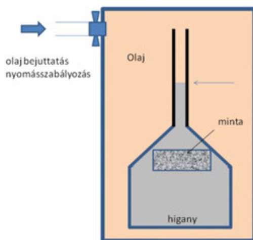
3.7. ábra. A higanytelítési módszer – mérési elrendezés. A telítési nyomást az olaj szabályozza.
