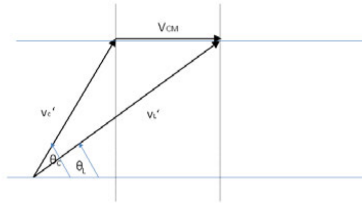
9.7. ábra. Tömegközépponti és laborrendszerbeli szórási szögek kapcsolata
