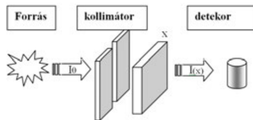
9.3. ábra. Makroszkópikus hatáskeresztmetszet mérése nyaláb kísérlettel
