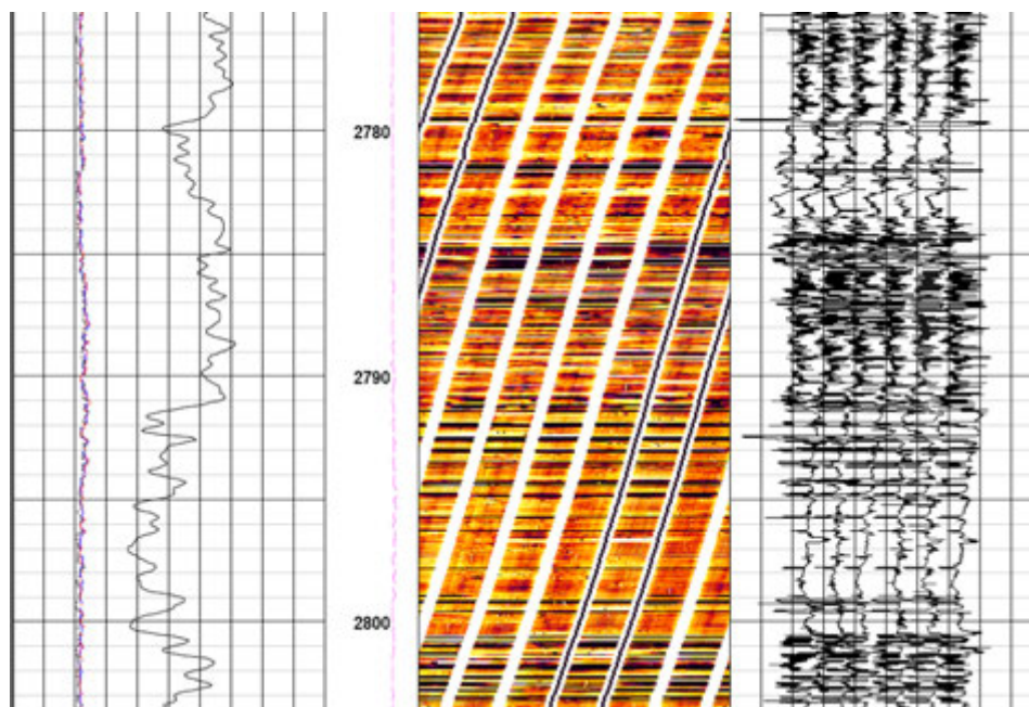
3.14. ábra. Lamináris agyag vezetőképésén alapuló lyukfal leképezésen (FMI szelvényen)
