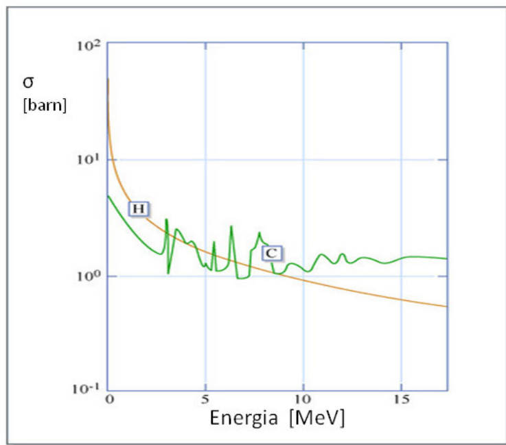
9.5. ábra. A hidrogén és szén neutron reakciókra vonatkozó totális hatáskeresztmetszetének energiafüggése. A csúcsok (rezonanciák) az abszorpciós hatáskeresztmetszeten jellemzők.
