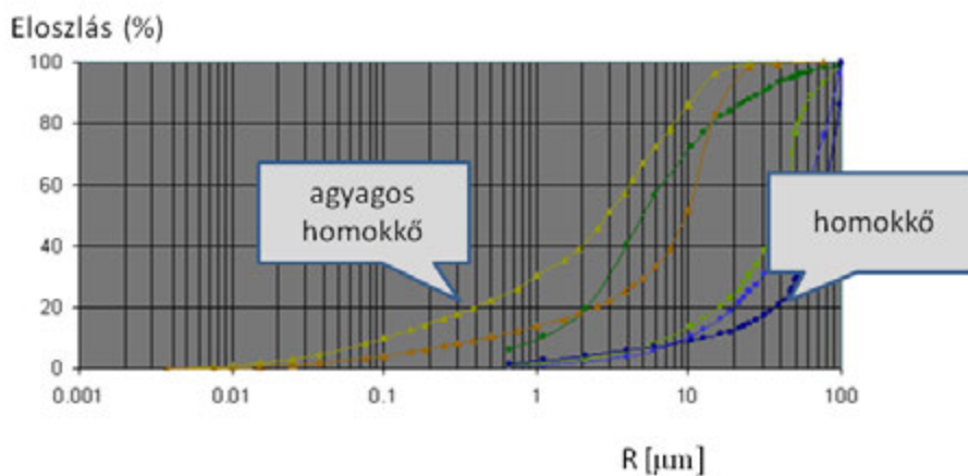
3.8. ábra. Tipikus higanytelítési mérésből származó pórustorok eloszlás görbék F(R)
