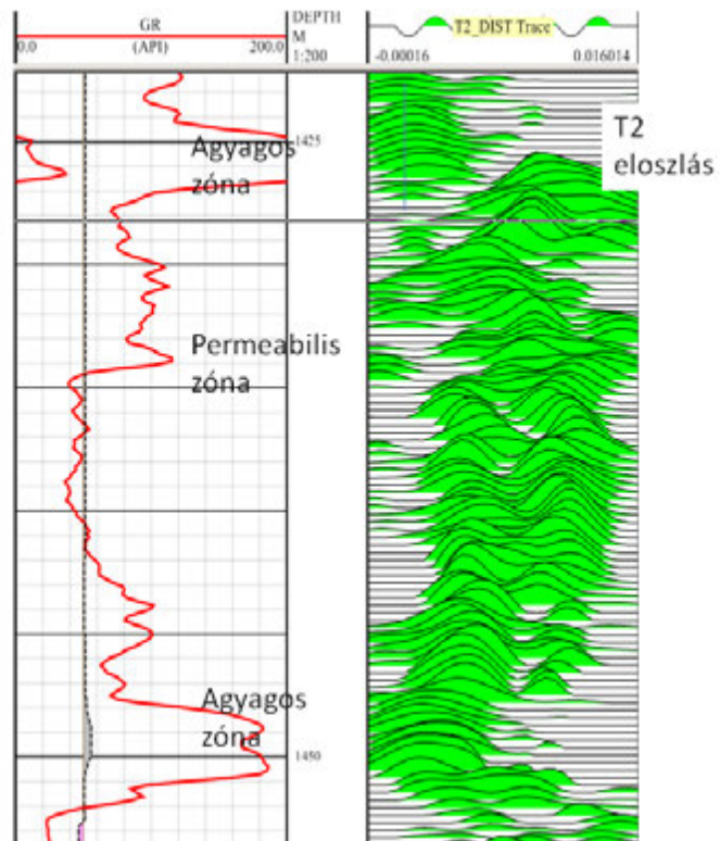
9.11. ábra. Fúrólyukban mért T_2 eloszlás görbék, jól mutatják a rövid relaxációs idővel jellemezhető agyagrétegeket, és a nagyobb T_2 -vel jellemezhető szabad pórusvizet. A tároló tetején a szénhidrogén is elkülönül.
