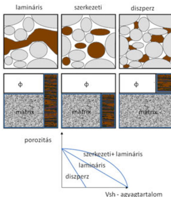
3.13. ábra. Agyagbetelepülés típusai
