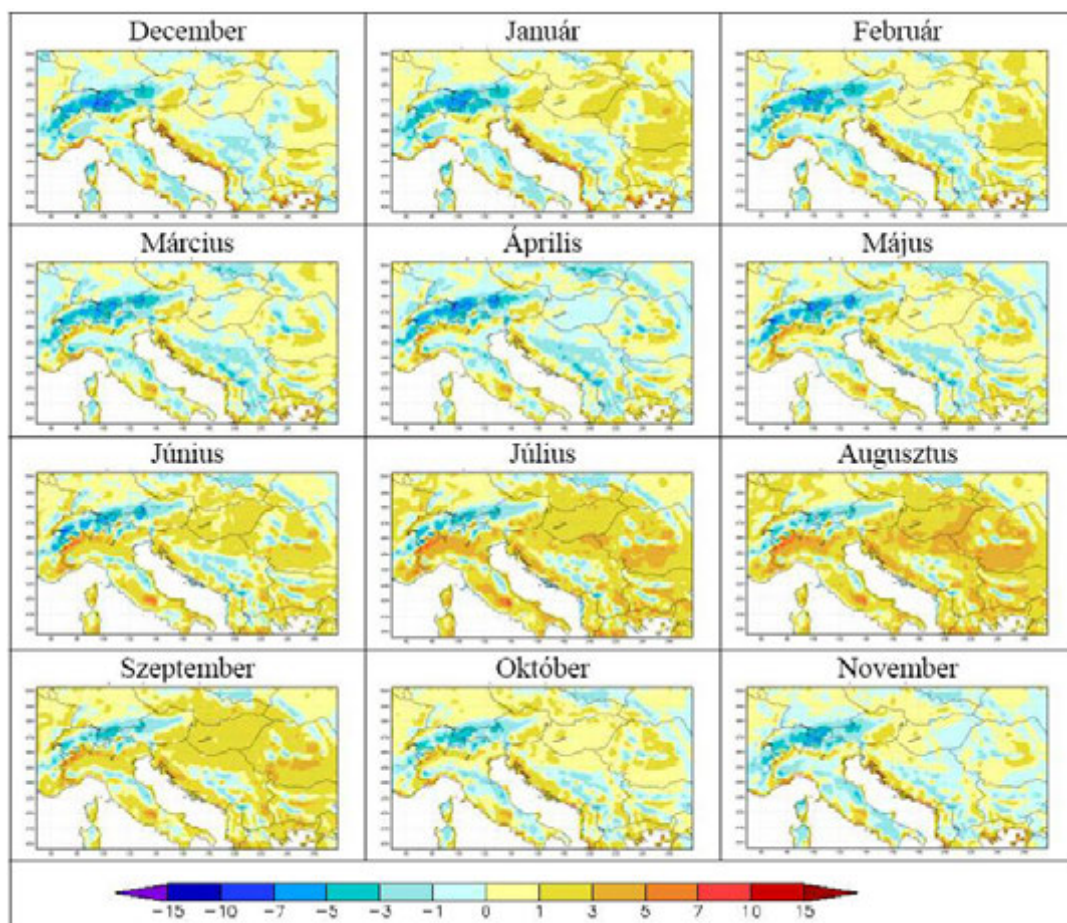
6.13. ábra. A PRECIS és a CRU adatbázis havi átlaghőmérsékleteinek eltérése (°C) a referencia időszakban, 1961–1990.
