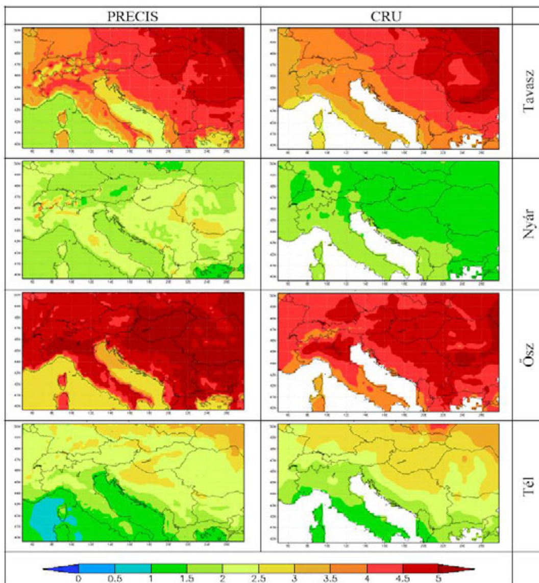
6.16. ábra. A PRECIS és a CRU adatbázis havi átlaghőmérsékleteinek évszakos szórása (°C) a referencia időszakban, 1961–1990.
