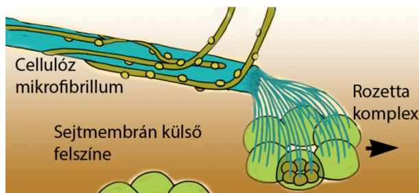
Rozetta komplex és a cellulóz mikrofibrillum szintézis.
