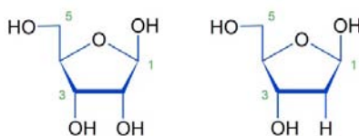
A ribóz és a dezoxiiribóz szerkezeti képlete.
