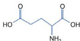
Glutaminsav (Glu; E) oldallánca savas
