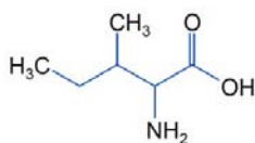
Izoleucin (Ile; I) oldallánca hidrofób
