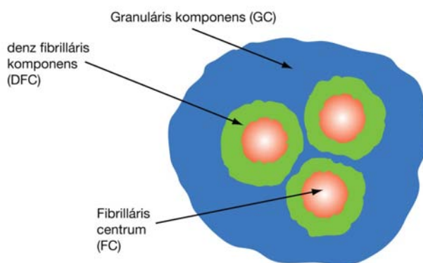
A nukleólusz komponensei
