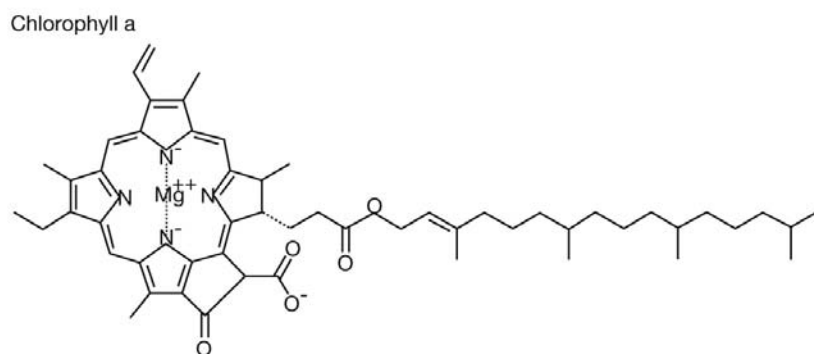
Klorofill a molekula szerkezete
