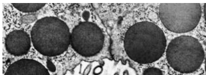
Váladékszemcsék a plazmamembrán alatt.
