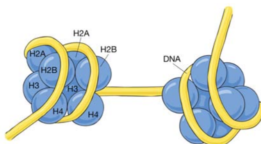
Nukleoszómkákra feltekert DNS szál
