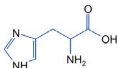
Hisztidin (His, H) oldallánca bázikus
