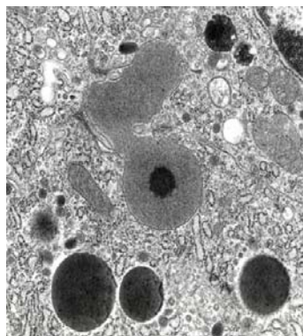
Váladékszemcsék a plazmamembrán alatt.
