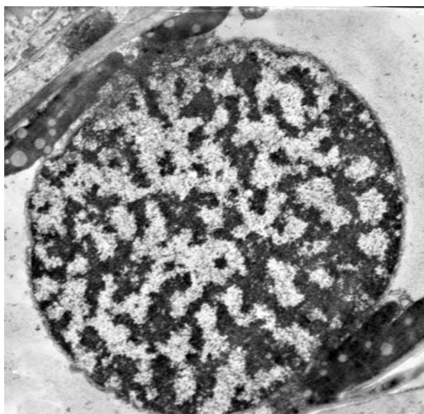
Heterokromatikus (sötét) és eukromatikus (világos) részek a sejtmagban
