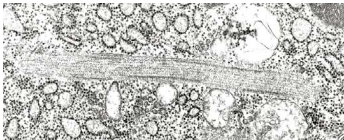
Mikrotubulus köteg. A taxol hatására a mikrotubulusok stabilizálódnak és kötegelődnek.
