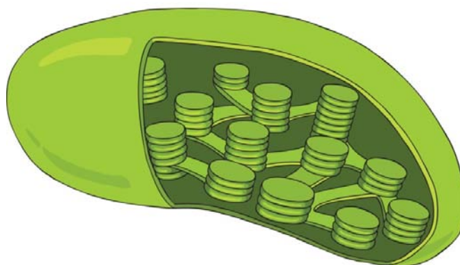
Kloroplasztisz tilakoid rendszere
