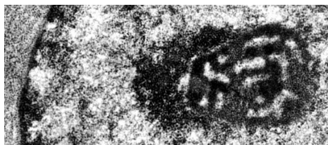
A sejtmagvacska metszete (TEM).
