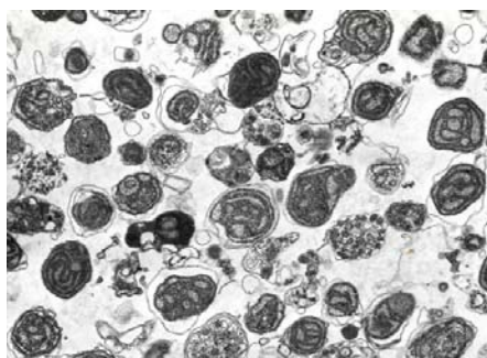
Autofág vakuólumok frakciója. Az eltérő elektrondenzitás az eltérő emésztettségi fokra utal.
