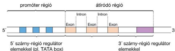
rRNS gén felépítése.
