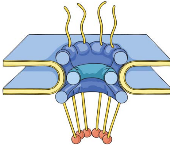
Magpórus komplex hosszszetszeti rajza.
