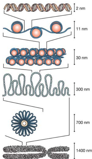
A kromoszóma hierarchikus szerveződése
