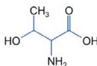
Treonin (Thr; T) oldallánca hidrofil
