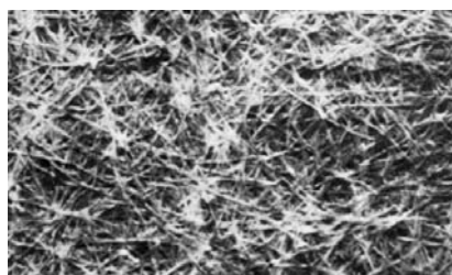
Elsődleges sejtfal felülnézeti képe (SEM fotó).
