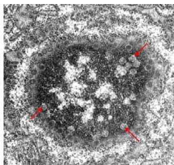
Magpórus (piros nyíl) érintőleges metszetének képe TEM fotón. A piros nyilak mutatják a magpórusok helyét.
