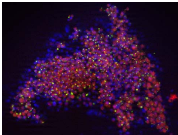
Ecetmuslica agyából készült metszet fluoreszcens festéssel (kék: DNS, piros: FIP200 fehérje, zöld: p62 fehérje jelölése; Nagy Péter felvétele).
