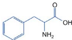
Fenil-alanin (Phe; F) oldallánca hidrofób
