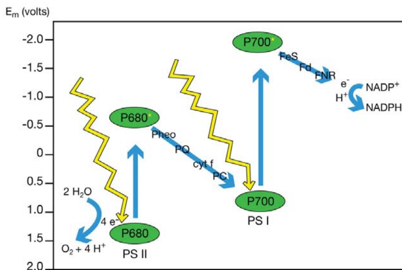
A fotoszintézis ún. Z-sémája az elektrokémiai potenciál függvényében.
