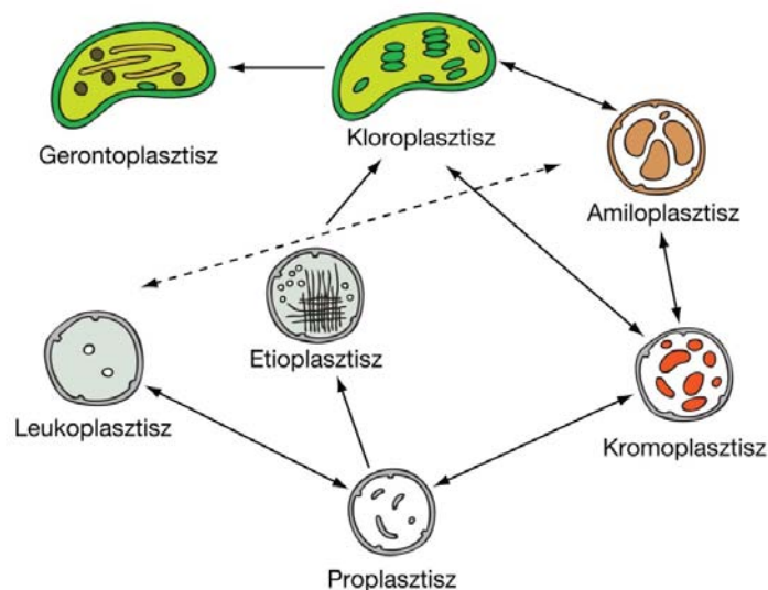
Plasztisz típusok, és egymásba alakulásuk
