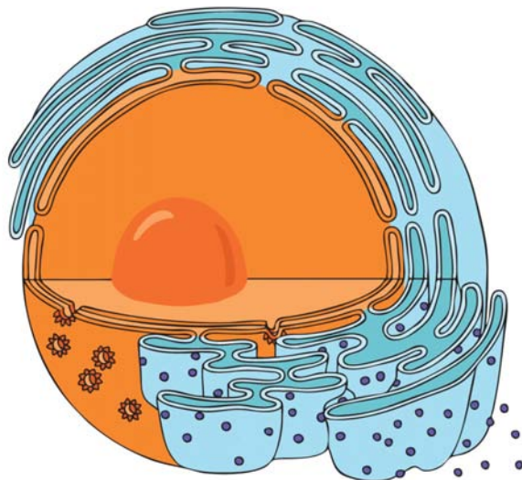
Sejtmag a sejtmagvacskával (sárga), és a maghártyához kapcsolódó ER-mal (kék)
