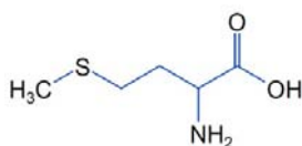
Metionin (Met; M) oldallánca hidrofób
