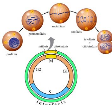
A sejtciklus általánosított sémája.
