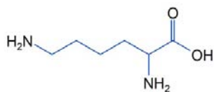
Lizin (Lys; K) oldallánca bázikus
